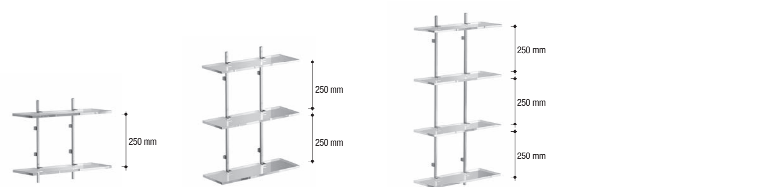
C452 C453 C454 Scaffale 2 piani 2-level shelf unit L. 450 H. 380 P. 162 mm Scaffale 3 piani 3-level shelf unit L. 450 H. 640 P. 162 mm Scaffale 4 piani 4-level shelf unit L. 450 H. 900 P. 162 mm
