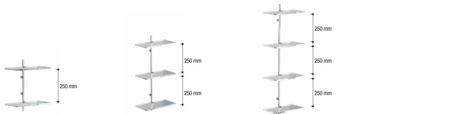
C442 C443 C444 Scaffale 2 piani 2-level shelf unit L. 300 H. 380 P. 162 mm Scaffale 3 piani 3-level shelf unit L. 300 H. 640 P. 162 mm Scaffale 4 piani 4-level shelf unit L. 300 H. 900 P. 162 mm
