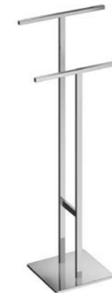
C477 Piantana lavabo Washbasin stand L. 330 H. 840 P. 200 mm Base 250 x 220 mm
